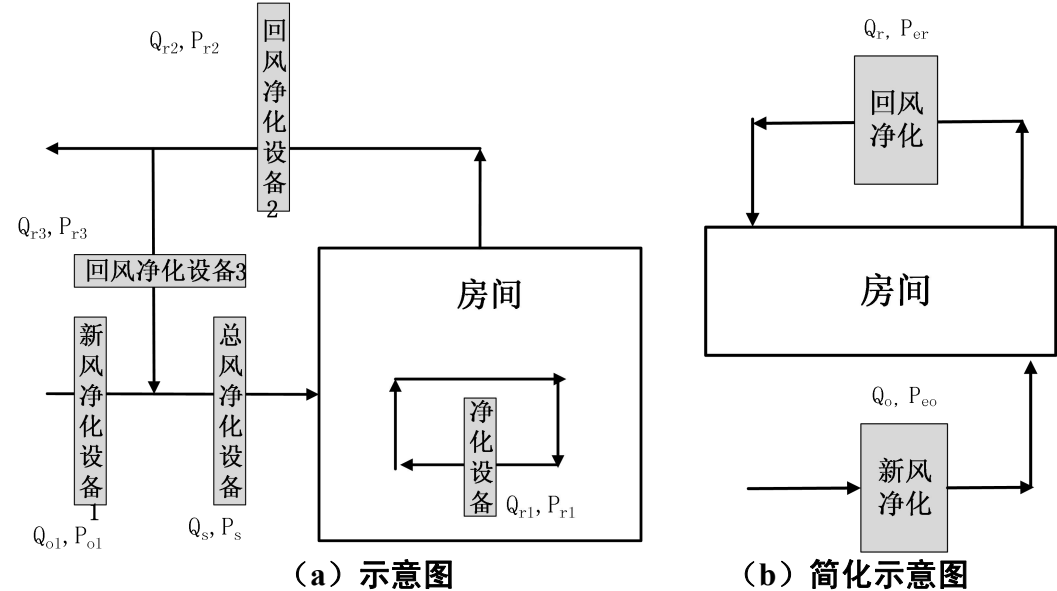
图 1 空气净化系统
